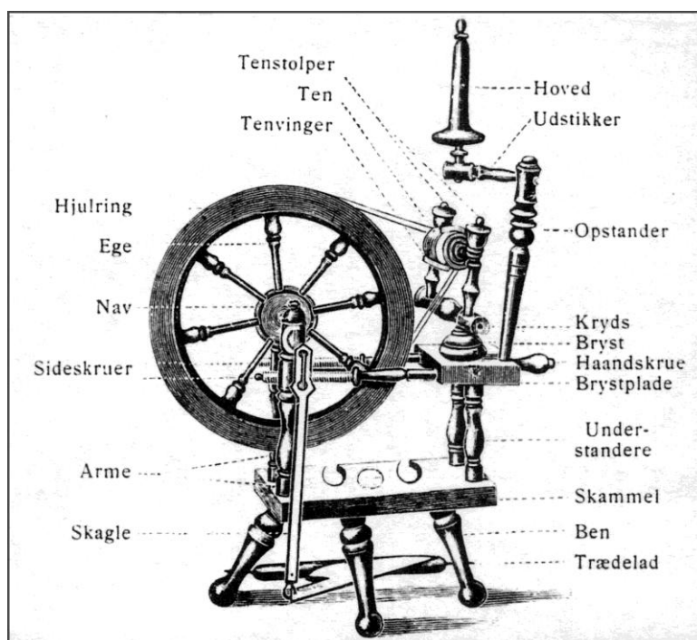
Spinderok fra Køgeegnen. H. F. Dalgaard, 1980.
